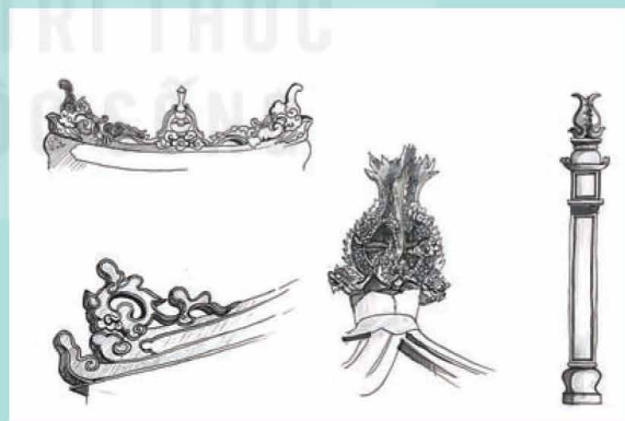
Bản vẽ các chi tiết kiến trúc trong Chùa Láng (4)
